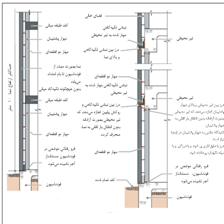
شکل ۵-۹ تکیه‌گاه‌ها جهت تحمل بار ثقیل نما
